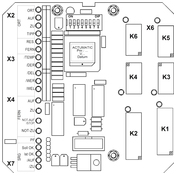
Bild 1: Logikplatine
